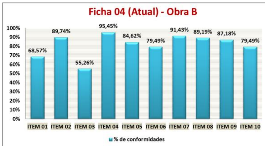
Figura 6 - Porcentagem das conformidades de cada item da Ficha 04 (atual) - Obra B
