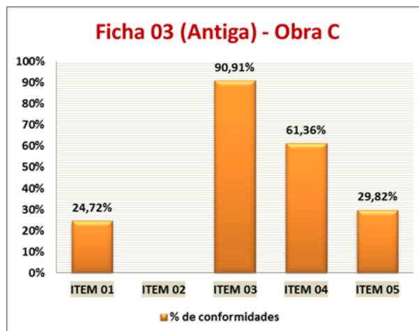
Figura 7 - Porcentagem das conformidades de cada item da Ficha 03 (antiga) - Obra C
