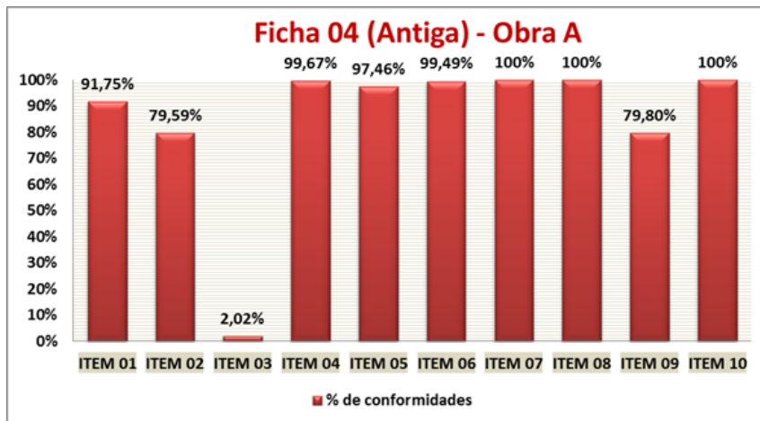
Figura 2 - Porcentagem das conformidades de cada item da Ficha 04 (antiga) - Obra A
