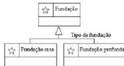
Fig. 9 - Generalização espacial.
