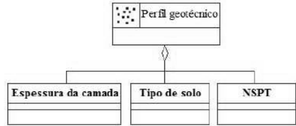
Fig. 7 - Agregação entre classes georreferenciada e convencional.
